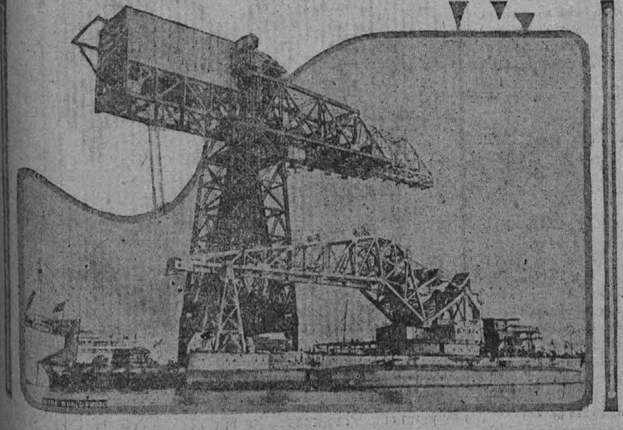
Na sliki vidite velikanskega nepremičnega 350-tonskega dvigača, ki se nahaja v Filadelfijski ladjedelnici. Takoj poleg pa se nahaja 312-tonski plavojoči dvigač, ki je sicer manjši, toda poseda skoro ravno toliko dvigalno moč kot prenepremični dvigač.
