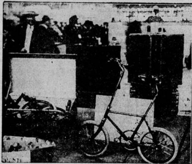
Zločivo kolo, ki je prišlo v promet v Parizu; zložiti ga je mogoče hitro v majhen kovček, kar je jako pripravno zlasti za shranjevanje.
