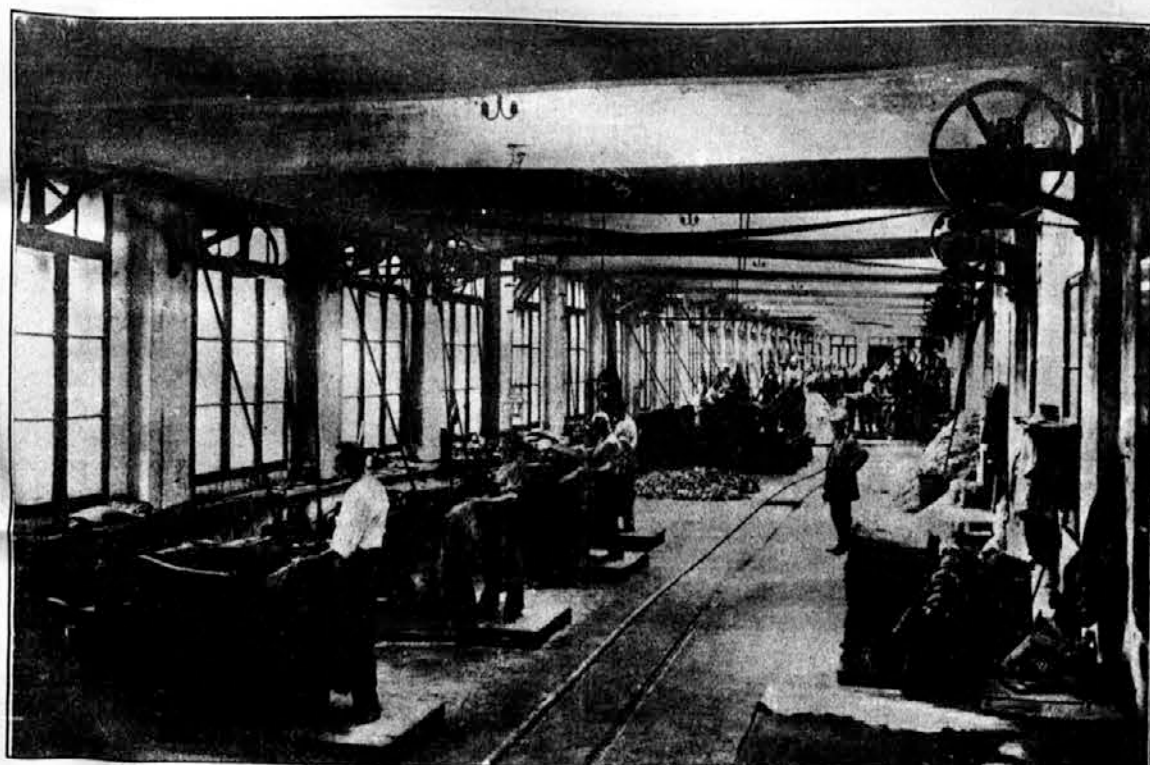
Iz notranjščine ljubljanske tovarne: Lužna delavnica in strojni oddelek usnjarske tovarne.
