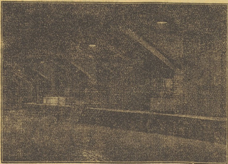
Beleuchtung einer Verladerampe durch Natriumdampfampfen der gleichen Type
