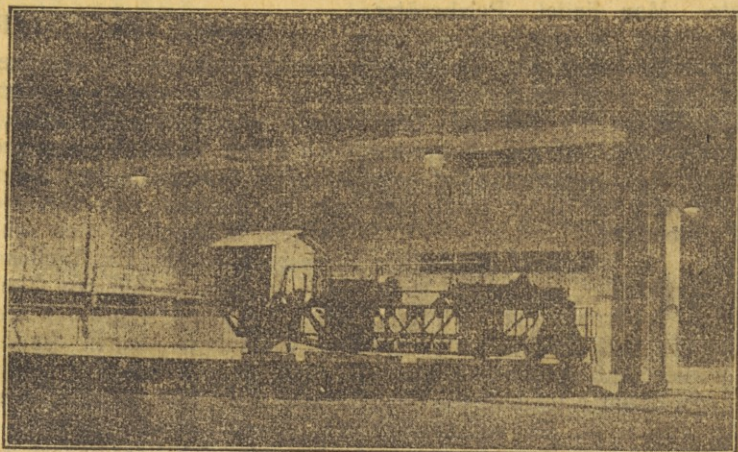
Beleuchtung des Rührwerkes für Schlamm im Vorratsbecken einer Zementfabrik durch zwei Natriumdampfampfen NA 300 (je 3000 Heiner-Lumen bei nur 68 Watt Leistungsaufnahme).
