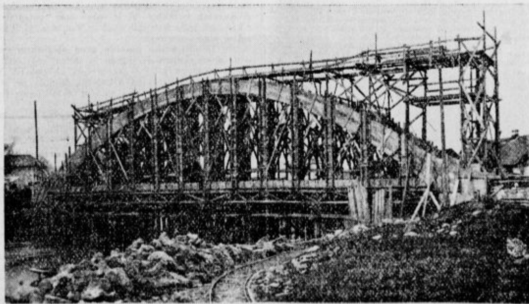
Pogled na novi most v Podpeči. Slika jasno kaže ves ogromni leseni opaž, v katerem se sedaj že utrjuje zabetonirani železobetonski lok in mostišče.
