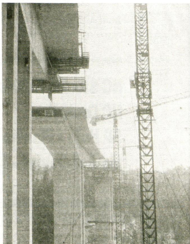
Viadukt Moste - gradbeno najbolj zahteven 444 metrov dolg objekt. Spojen mora(!) biti (tudi zaradi načina gradnje) julija oziroma avgusta letos, "prevozen" pa v začetku novembra...
