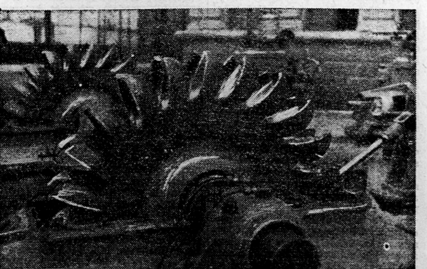
Delovni kolektiv Litostroja bo pokazal svoje uspehe pred Narodnim domom v Ljubljani. Na sliki gonilno kolo za Peltonovo turbino
