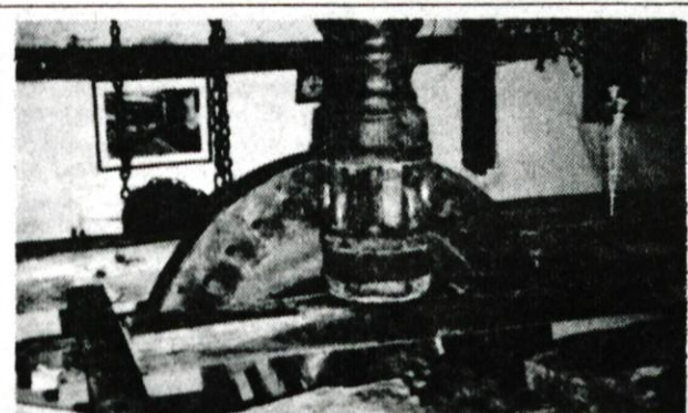
Pogonsko kolo za mongo - likalnico v nekdanji Pirčevi barvarni v Kranju. Foto: Mirko Križnar
