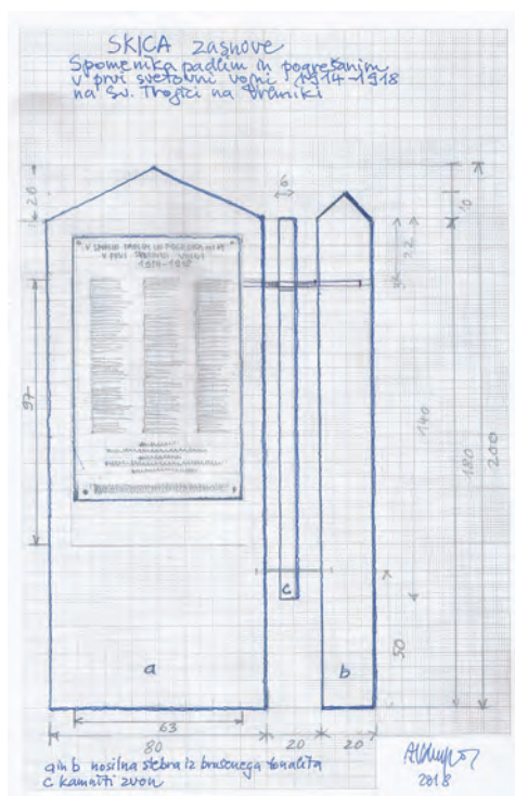
Spomenik padlim in pogrešanim vojakom v 1. svetovni vojni na Sv. Trojici na Vrhniki; levo skica umestitve v prostor, desno skica pogleda. Risba: Alenka Vidrgar, 2018.
