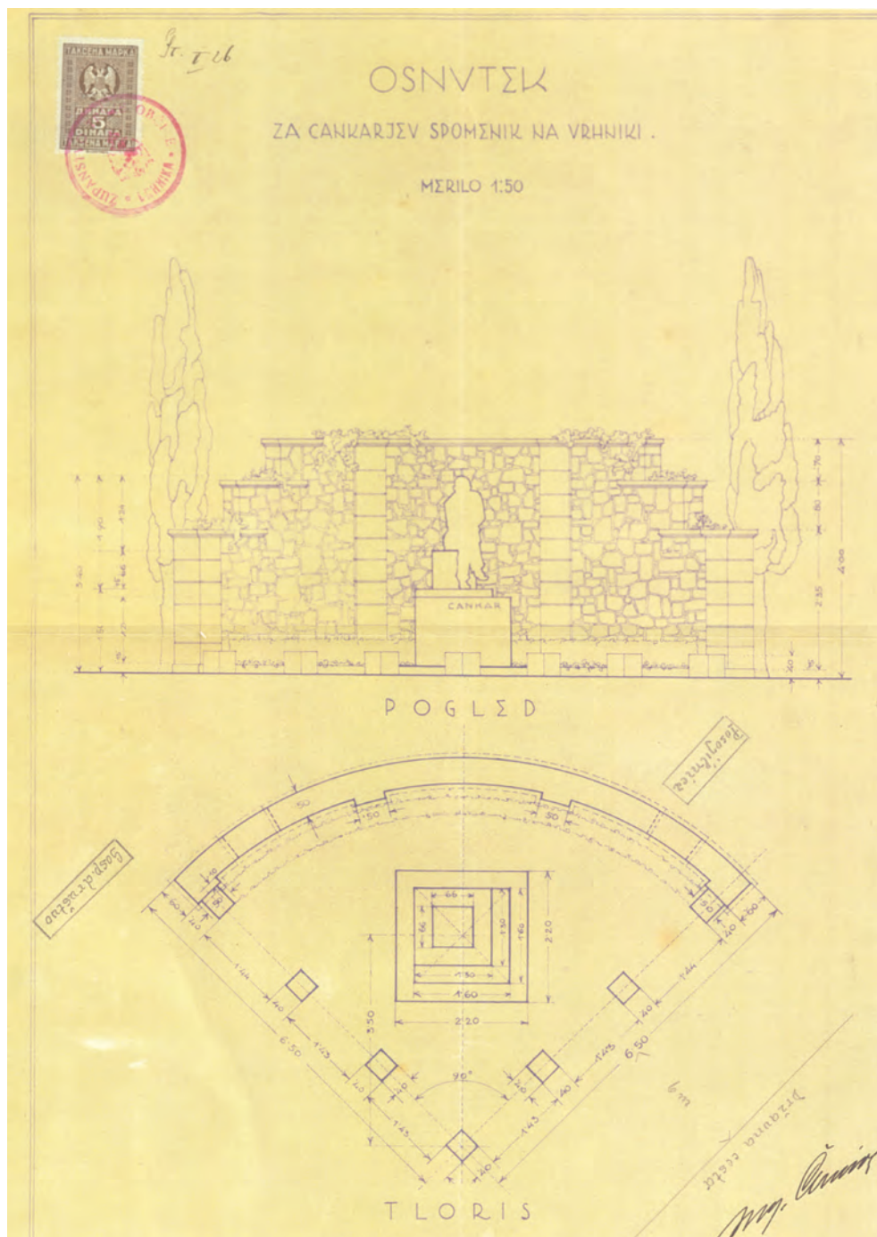
Osnutek za postavitev spomenika je izdelal ing. Črničev. (Zgodovinski arhiv Ljubljana, sign.: VRH 2, gradbene zadeve 14, a. e. 1520)
