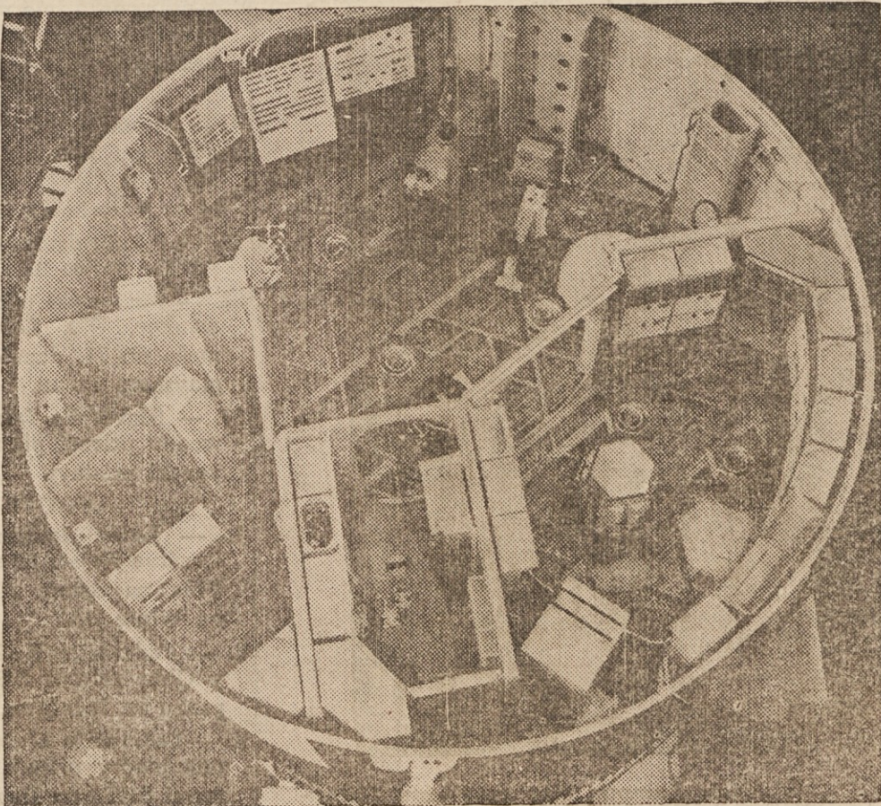
TESNO BIVALISCE IN DELAVNICA — Slika kaže počesni prerez modela vesoljske postaje, kot jo bodo ZDA prihodnje leto poslale na kroženje okoli Zemlje. V njej je prostor za bivanje, pa tudi za delo in opravljanje poskusov. V vesoljski postaji bodo delale posadke treh članov po 28 do 56 dni.
