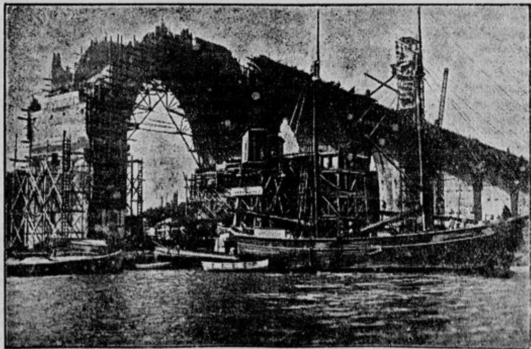
Največji železniški most na Švedskem, ki ga gradijo v Stockholmu in bo gotov šele leta 1929. — Dolg bo 750 metrov, a pod njegovimi oboki bodo lahko plavale največje ladje.
