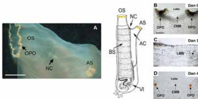
Slika 2. Anatomija Cione . OS – Oralni (dotekalni) sifon, AS – atrialni (izmetalni) sifon, NC – možgani (živčni vozli), BS – škvržna košara, VI – drobovina (želodec, srce, gonade), AC – kloaka. A. Pogled od zgoraj na distalni del telesa. OPO – oranžno pigmentirani oceli. Merilo: 10 mm. B. Rob intaktnega sifona pri mladem osebkju. Lobe – mišična krpa, CMB – krožna mišična vlakna. Merilo: 1 mm. Merilo je enako na slikah C. in D. C. Rob odrezanega vrha sifona en dan po odstranitvi. LMB – vzdolžna mišična vlakna. D. Rob sifona med regeneracijo četrty dan po odstranitvi prvotnega sifona.
