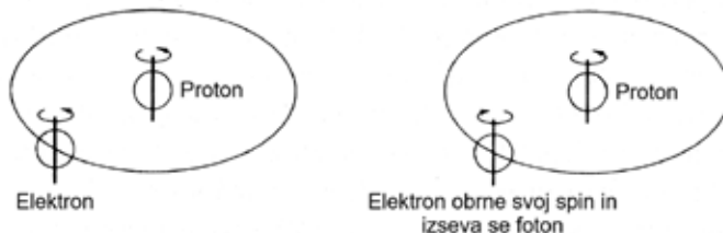
Slika 6: Nastanek vodikove spektralne črte pri 21 cm valovne dolžine. Na levi sliki imata proton in elektron istosmerna spina, na desni pa je spin elektrona nasproten spinu protona.
