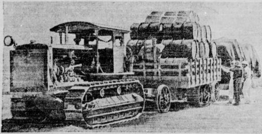
Italijanski tovorni avtomobili imajo v Abesiniji namesto koles take »gosenčje verige«, s katerim se poganjajo naprej po težavnem ozemlju.
