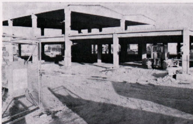
Market v Slovenskih Konjicah zgrajen po našem montažnem sistemu
