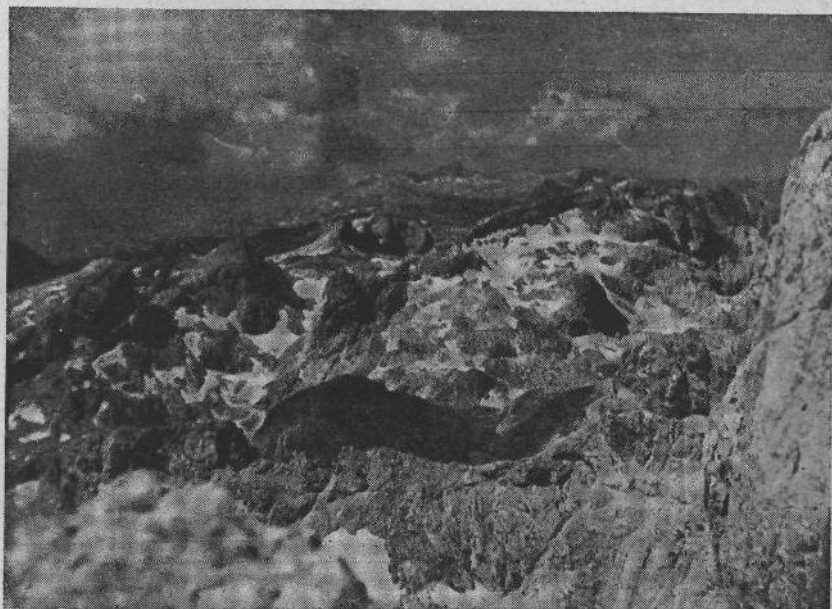
Sl. 5. Kanjavec, Hribarice, Velska dolina, v ozadju Krn 17. avgusta 1951
