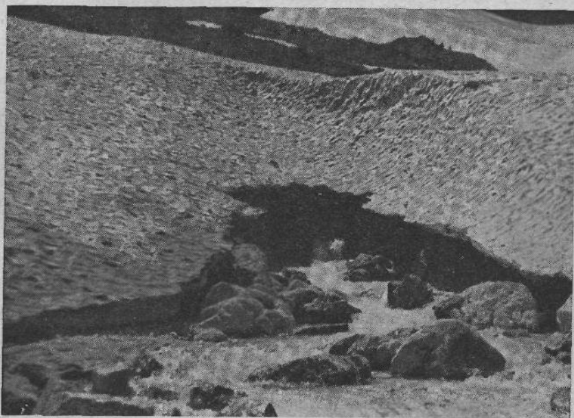
Sl. 3. Vodna vrata na koncu glavnega snežišča ob izviru Vratske Bistrice 12. avgusta 1951
