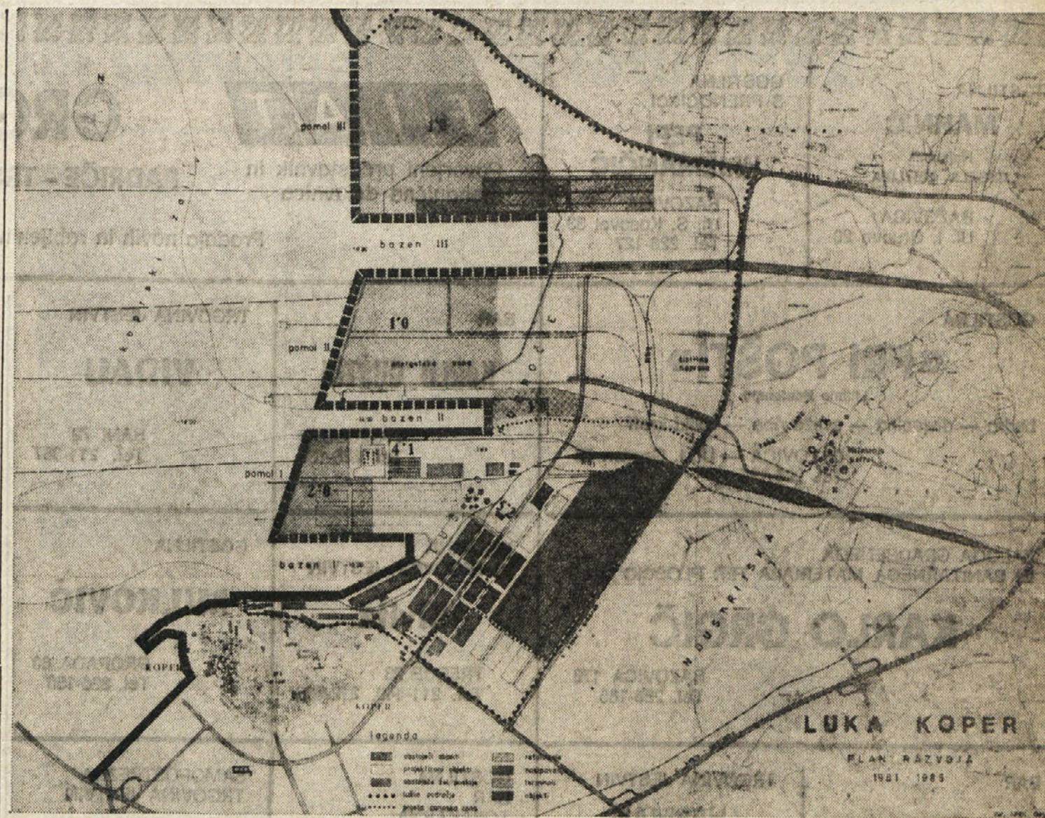
Situacija dolgoročnega razvoja luke in energetske industrijske cone (obstoječi objekti in predvidene gradnje)
