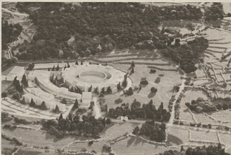
Maketa sinhrotronskega svetlobnega pospeševalnika
