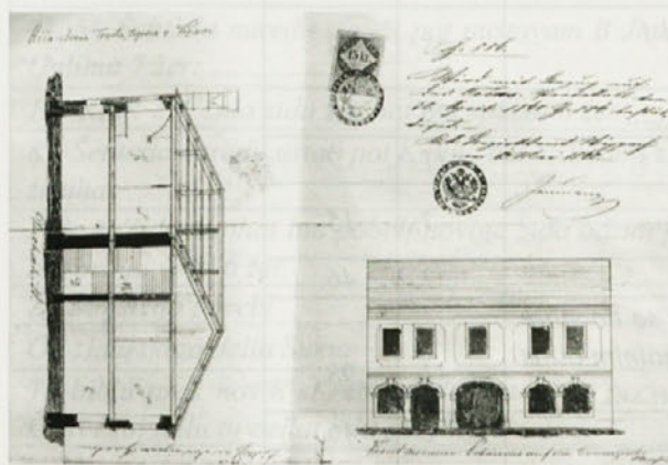
Del načrta za prezidavo in dozidavo hiše, ki ga je leta 1860 naredil po naročilu Janeza Trosta znameniti zidarski mojster Miha Blažko iz Lokavca.
