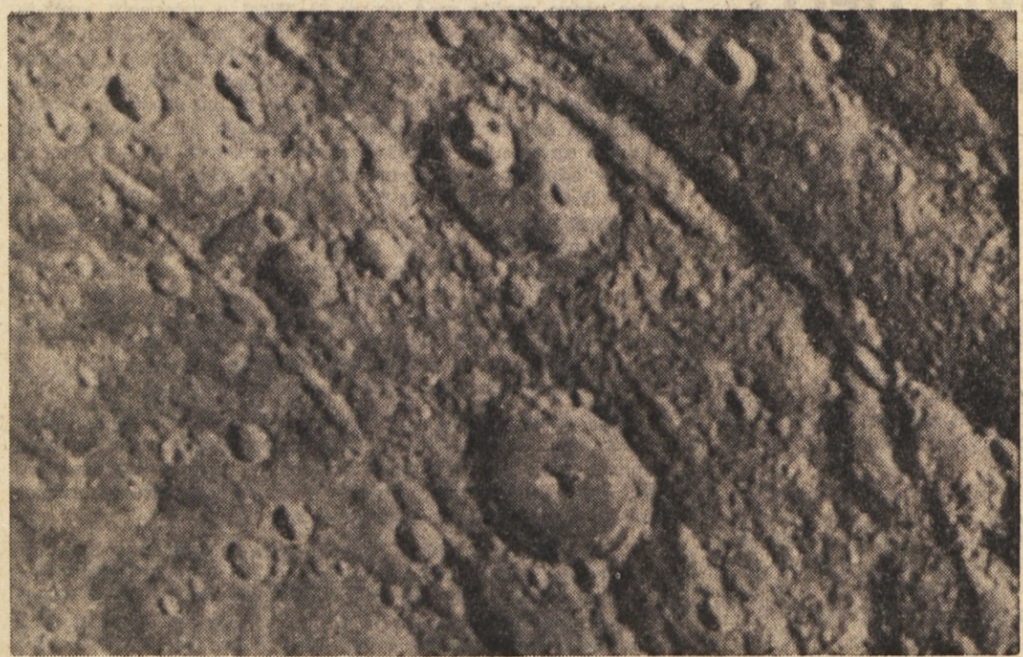
Merikurova površina, kot jo je posnela ameriška avtomatska sonda mariner
