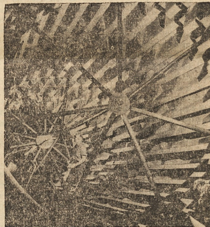
MLIN NA NOGE? — Nekdaj so posebno v nekaterih delih Azije uporabljali mlin na noge. Vrtel se je s tem, da so njegovi gonjači stopali od stopnice na stopnico. Tale slika bi lahko kazala nekaki ogromni mlin te vrste, dejansko pa je to le velikanski boben za sušenje fosfatnih produktov, kot jih izdeluje Allis-Chalmers.
