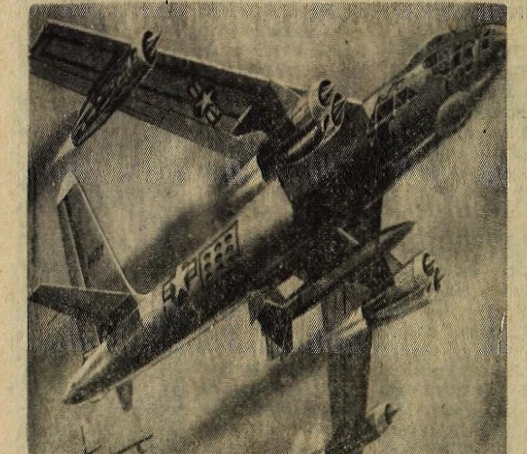
Ameriško letalo Boeing B-47 je namenjeno za nosilca raket; naša slika prikazuje letalo, ki nosi takšno raketo. Rakele lahko izstrelijo v horizontalnem in v navpičnem letu
