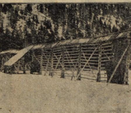
Od leve na desno: vezani kozolec (toplar) v Ravnem na Zgornjem Jezerskem; stegnjeni kozolec z lopo v Zgornjesavski dolini; primitivnejša oblika stegnjenega kozolca s Koprivnika nad Bohinjem; prislonjeni kozolec na Zgornjem Jezerskem
