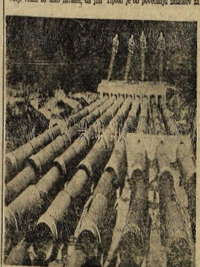
Vzhodnoslovaška elektrarna pri Hohenwaru, ki jo bodo zgovalili do 1963. leta. Vodo iz reke Saale bodo v nočnih urah črpali v umetno jezero. V kritičnih urah jo bodo spustili po ceveh do turbin
