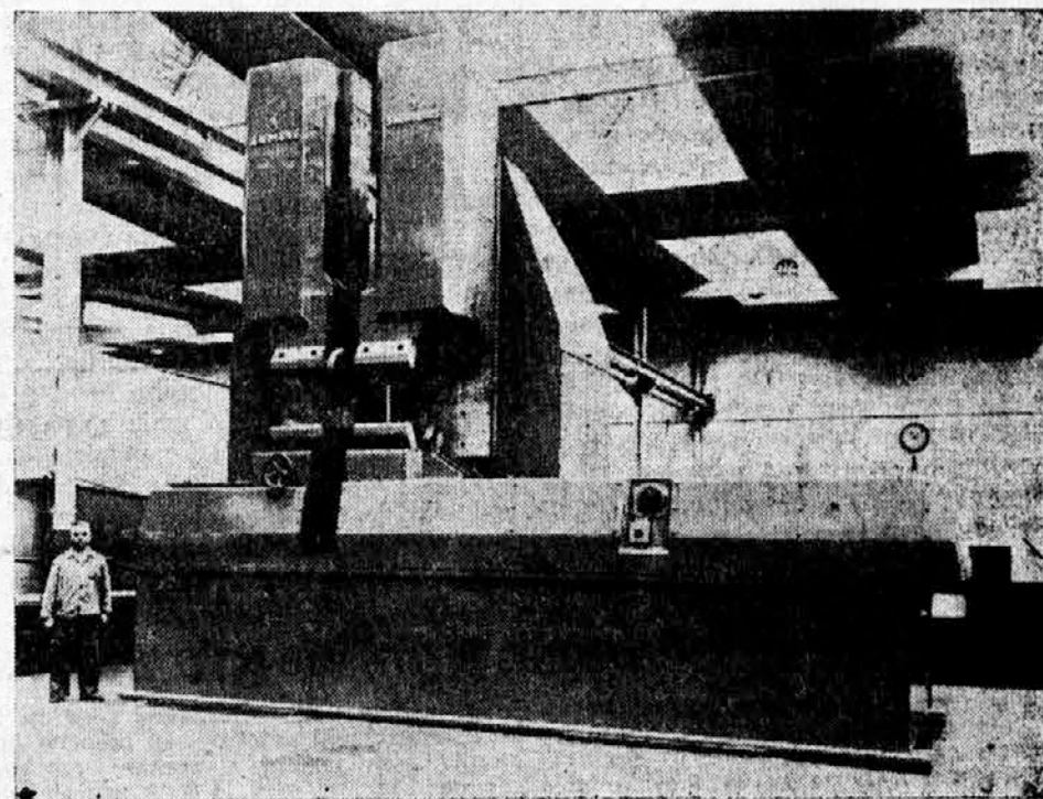
Največja avtomatična varilnica na svetu. Postavila jo je tvrdka Siemens-Schuckert v Nürnbergu
