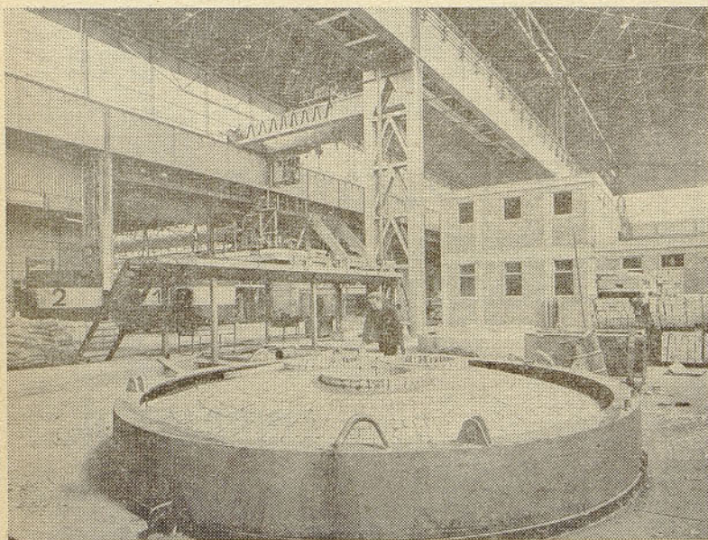
Obzidava pokrova elektropeči v Jeklarni II
