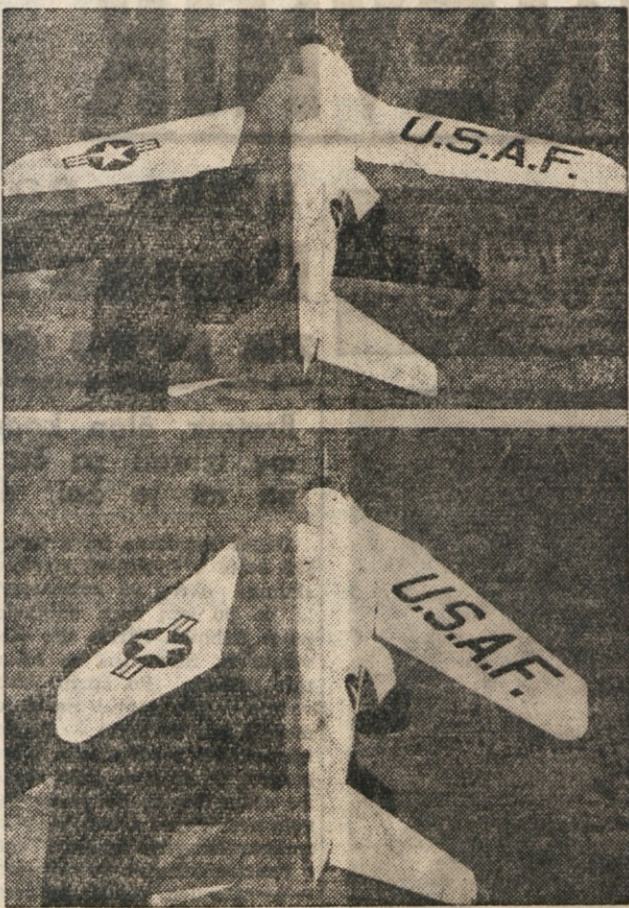
Prvo ameriško letalo vrste X-5 s krili, ki jih letalec med poletom lahko prekriva po potrebi nazaj ali naprej. Med vzletom in pri spuščanju so njegova krila pomaknjena naprej, ko leti z največjo brzino pa nazaj (spodnja slika).
