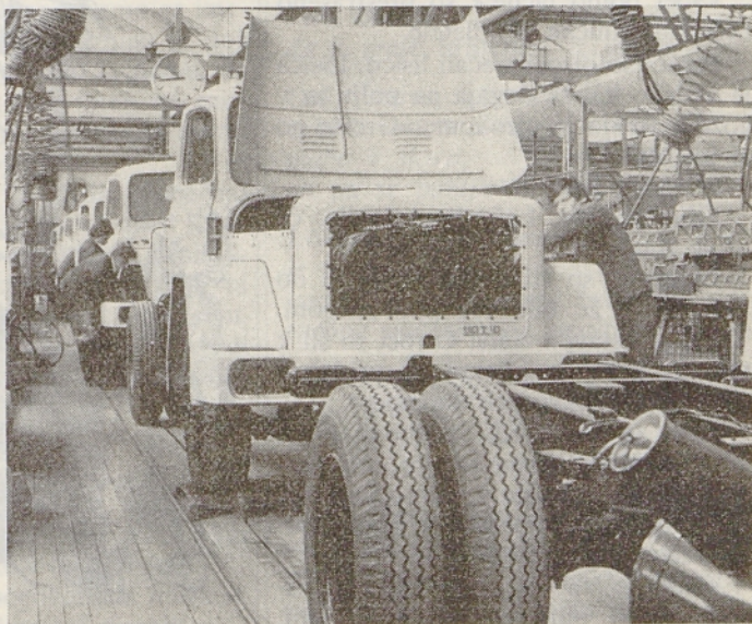
Montaža vozil v TAM.
