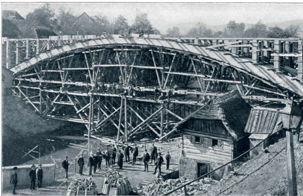
MOST ČEZ DOBLIČANKO PRI ČRNOMLJU (MED ZGRADBO).
