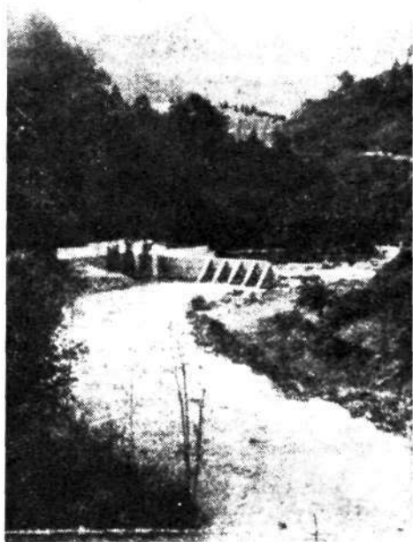
Podrt betonski jez za električno centralo na Fužinah po povodnji 18. junija 1925.
