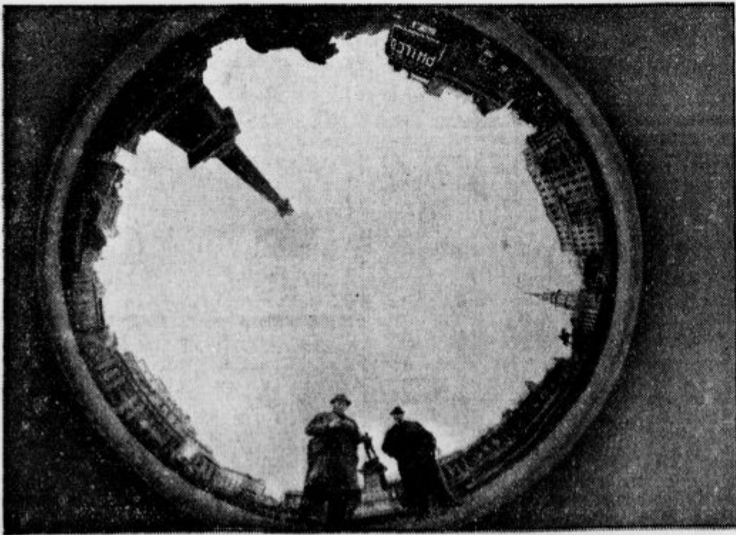
Fotografski aparat, ki svet drugače gleda. Anglež Robin Hill je iznašel kamero, ki ob enem vidi na vse strani. Elektromagnet proži zaklop aparata. Na naši sliki vidimo fotografijo sredi Londona.
