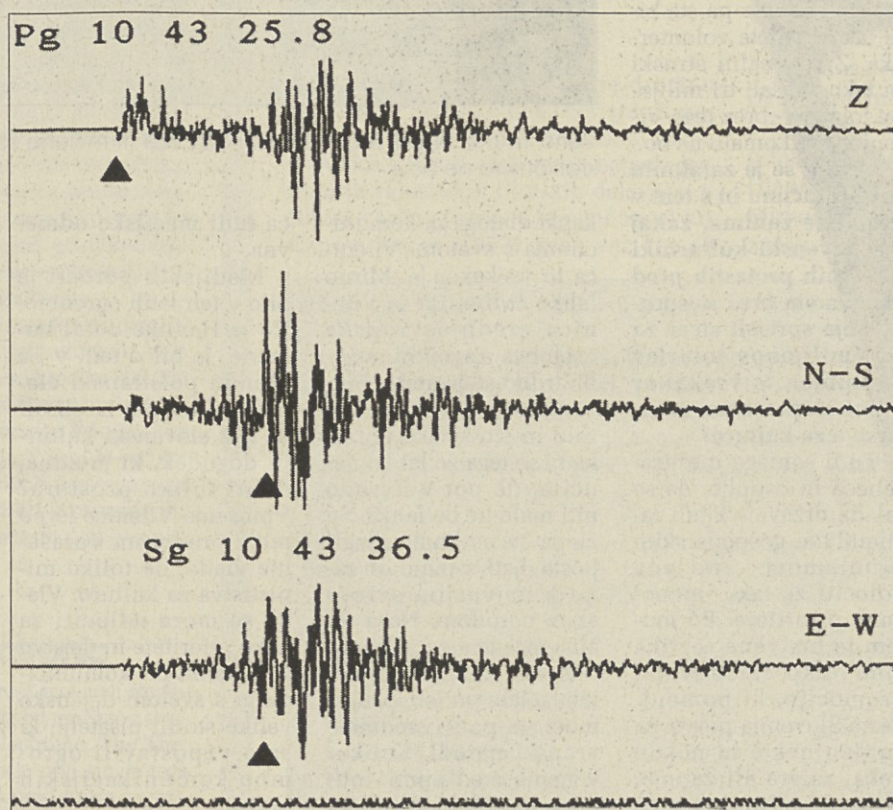
Zapis treh komponent potresa 29. maja 1993 ob 10. uri 43 minut z epicentrom na obrobju Bele Krajine
