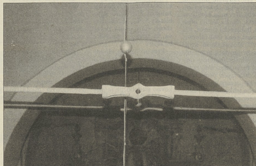
Vgrajena potresna vez v cerkvi Sv. Vida v Gribljah
