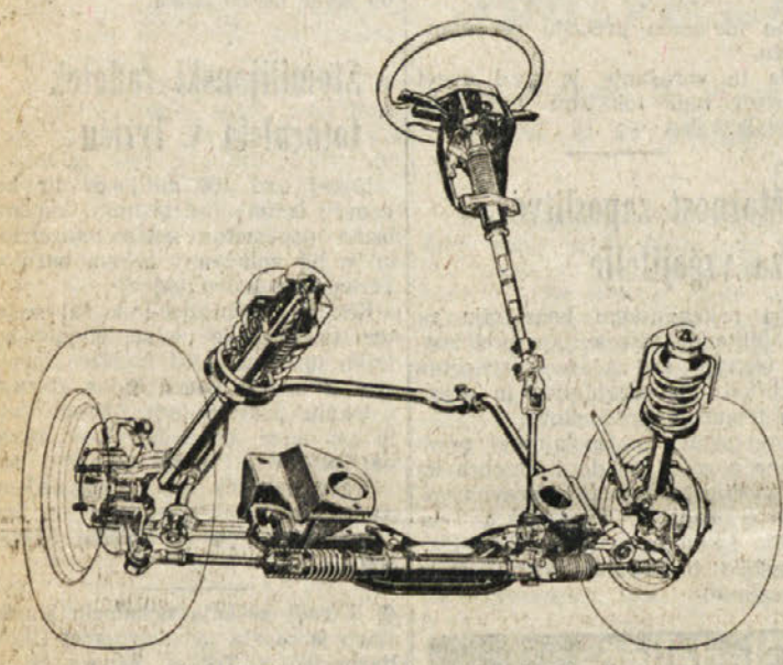
Sierra ima spredaj McPhersonovo premo in stabilizator obrnjen nazaj
