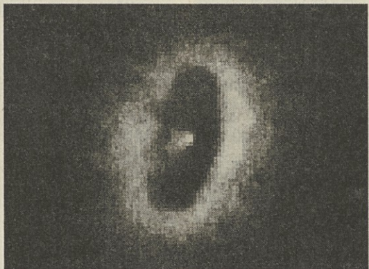
Hubblova širokokotna kamera je slikala črno luknjo v področju galaksije NGC 4261.
