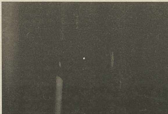
Modri blisk iz zračnega mehurčka v vodi utripa s frekvenco zunanjega zvočnega polja (SA)
