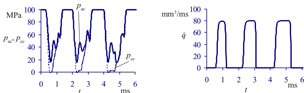
Sl. 9. Karakteristike vbrizgavanja pri trostopenjskem vbrizgu ( d_{rv} = 0,3 \text{ mm} , 3/2 sv)
