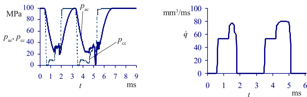
Sl. 10. Karakteristike vbrizgavanja pri dvostopenjskem vbrizgu ( d_{hv} = 0,2 \text{ mm} , 3/2 sv, h_{nl} = 0,07 \text{ mm} )
