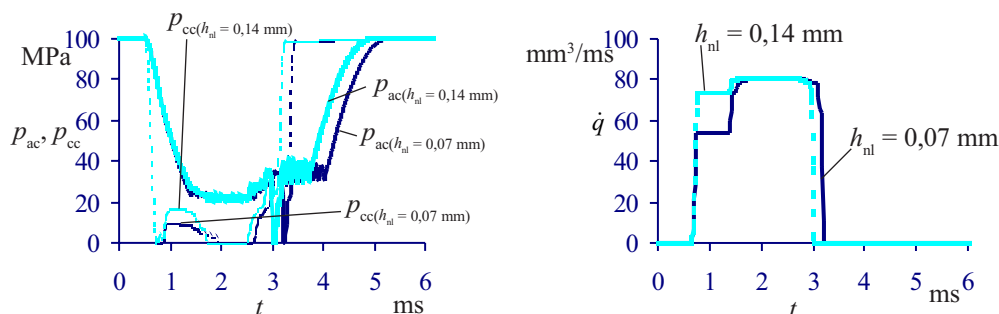
Sl. 8. Vpliv preddviga igle vbrizgalne šobe ( d_{hv} = 0,02 \text{ mm} , 3/2 sv)
