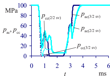
Sl. 6. Vpliv različnih tipov solenoidnih ventilov ( d_{rv} = 0,3 mm) Fig. 6. The influence of the different types of the solenoid valves ( d_{rv} = 0,3 mm)
