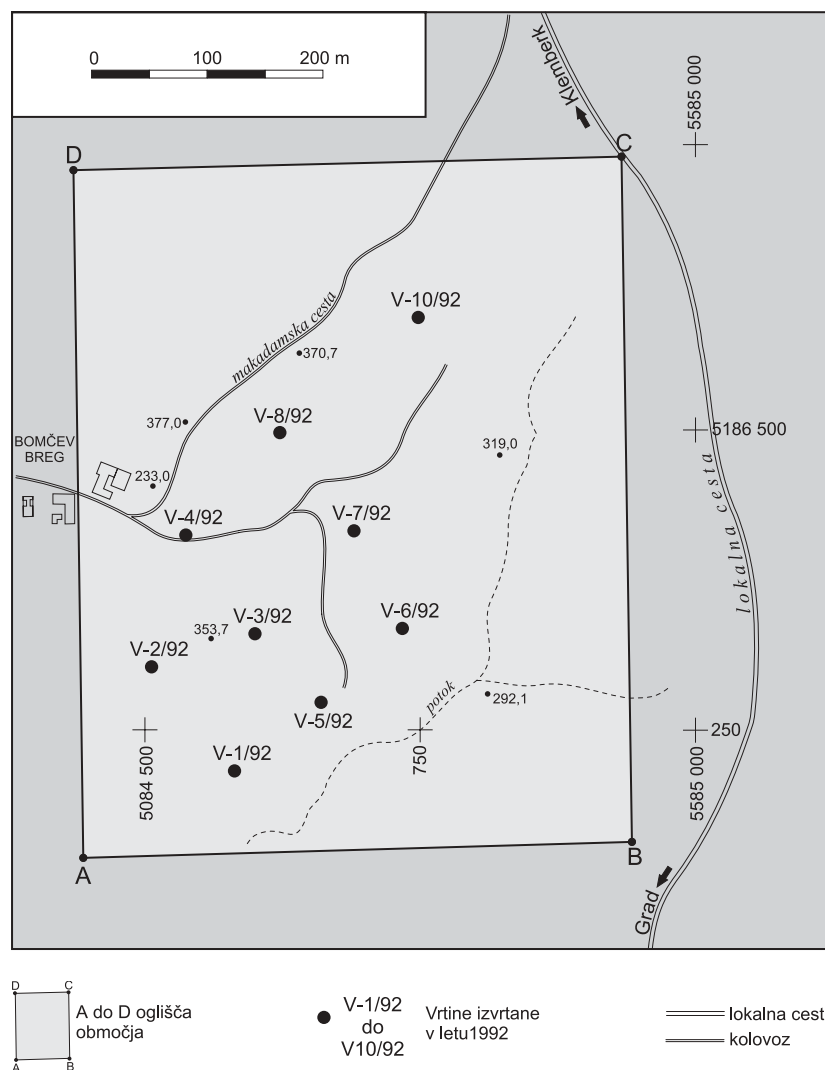
Slika 3. Območje raziskav glin s situacijami vrtin na lokaciji Bomčev Breg (po Stregarju, 1992)
