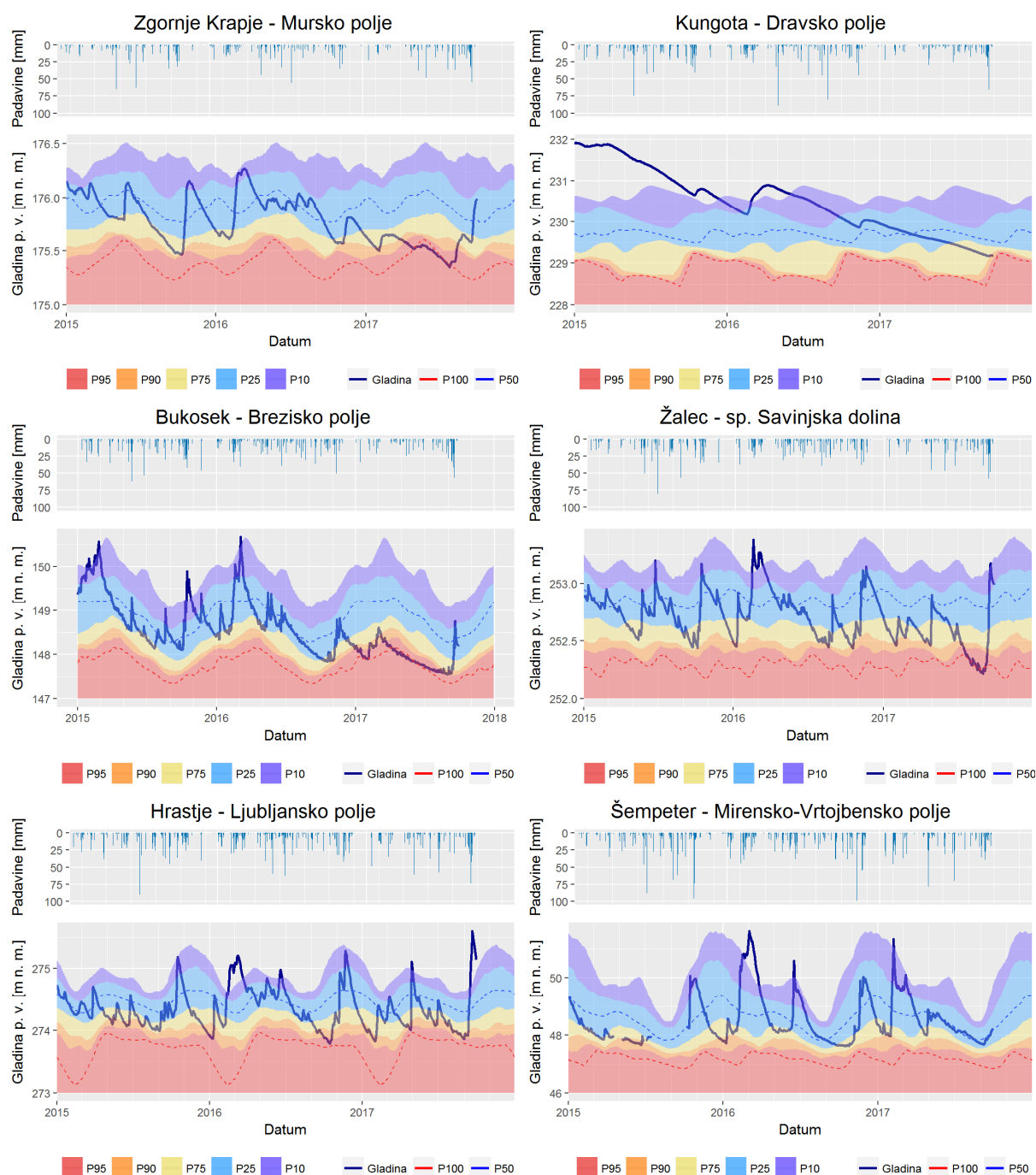
Slika 5. Srednje mesečne gladine podzemnih voda (m.n.v.) med letoma 2015 in 2017 v primerjavi z značilnimi percentilnimi vrednostmi gladin primerjalnega obdobja 1981–2010, zglajenimi s 30-dnevnim drsečim povprečjem Figure 5. Monthly mean groundwater level (m a.s.l.) between years 2015 and 2017 in relation to percentile values for the comparative period 1981–2010, smoothed with 30-day moving average
