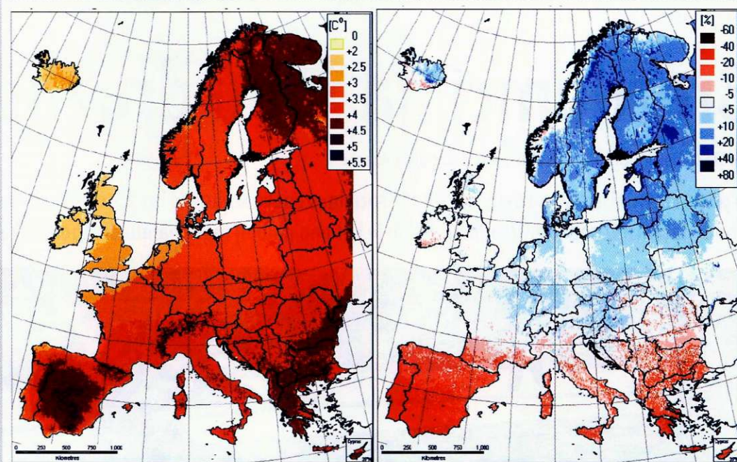
Sprememba povprečne letne temperature do konca tega stoletja v Evropi
