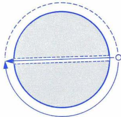
Slika 3. Umetni satelit, ki bi krožil okoli Zemlje v majhni višini, bi potreboval do nasprotni točke enak čas kot telo, ki bi padlo mimo središča Zemlje.
