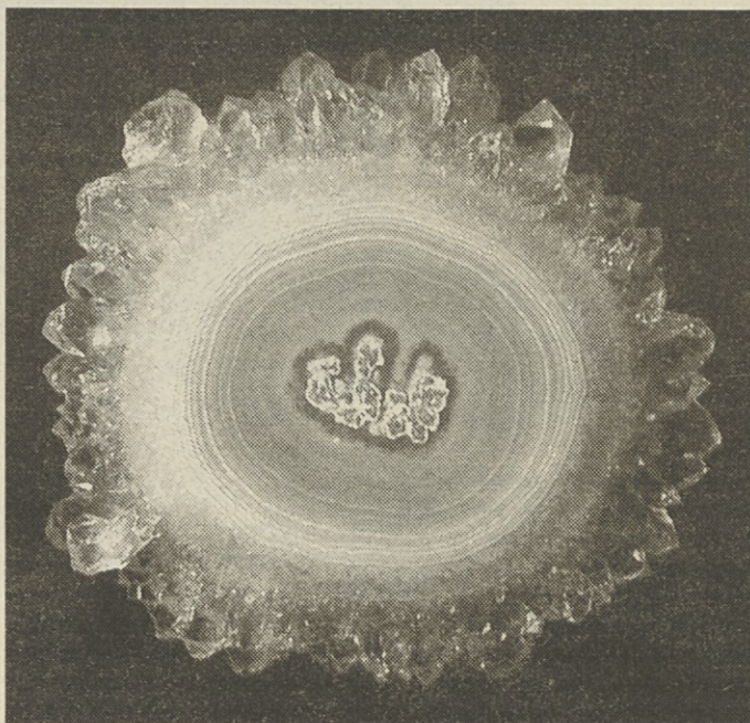
Ahat (v sredi), ki ga obdaja ametist
