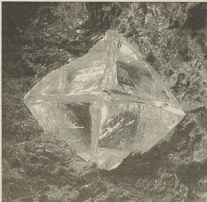
Kristal diamanta v kamnini
