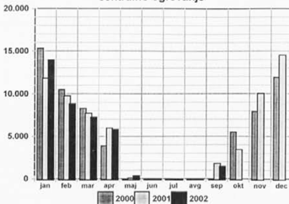
Proizvodnja toplote za centralno ogrevanje
