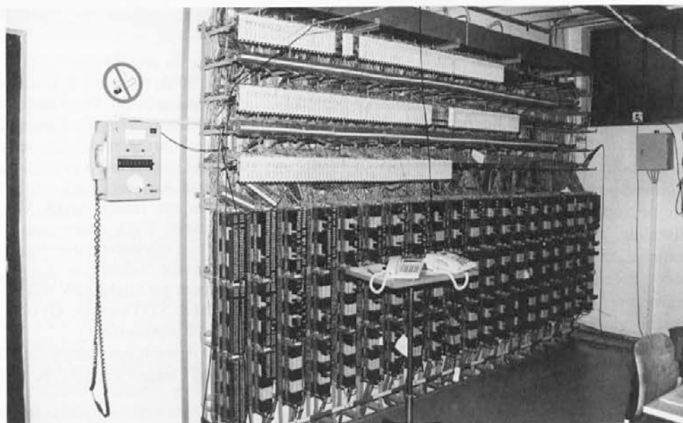
Del nove Telekomove centrale CENTREX
