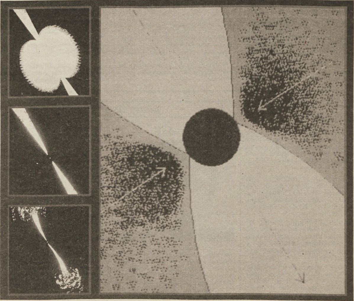
Hipotetična struktura črne luknje v vesolju (Iz kataloga pariške razstave »L'immaginario scientifico«)
