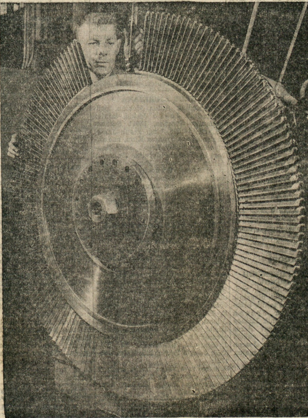
ZA PARNO TURBINO — Tehnik namešča lopatice na kolo za veliki parni turbinski generator. Vsaka lopatica je nameščena posebej in pritrjena.
