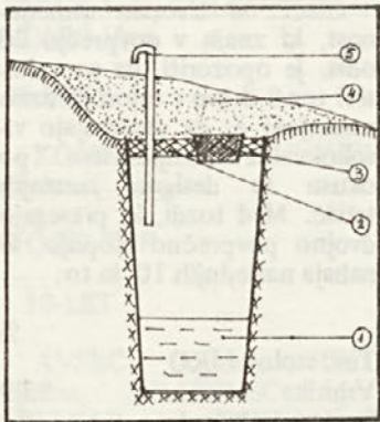
Zaščita vodnjaka: 1. vodnja, 2. betonska plošča, 3. odprtina za vhod, 4. zaščitna plast zemlje, 5. cev za prezračevanje.
