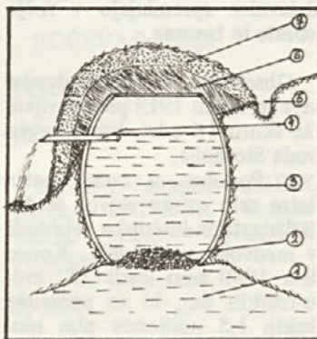
Improvizirana kaptaža: 1. talni izvir, 2. pesek, 3. sod, 4. kos cevi, 5. kanal, 6. plast gline, 7. ruša.
