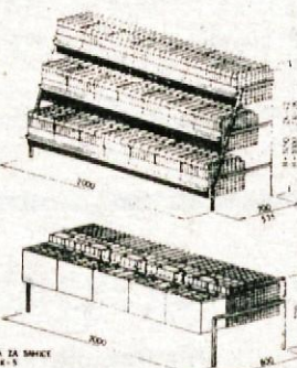
ETAŽNA KLETKA ZA ZAJCE
