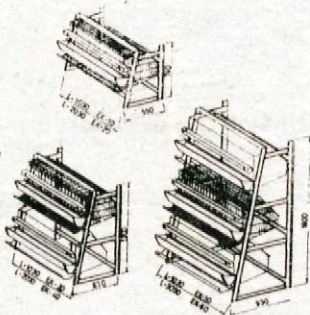
ETAŽNA KLETKA ZA KOKOŠI NESNICE IN BROJLERJE
