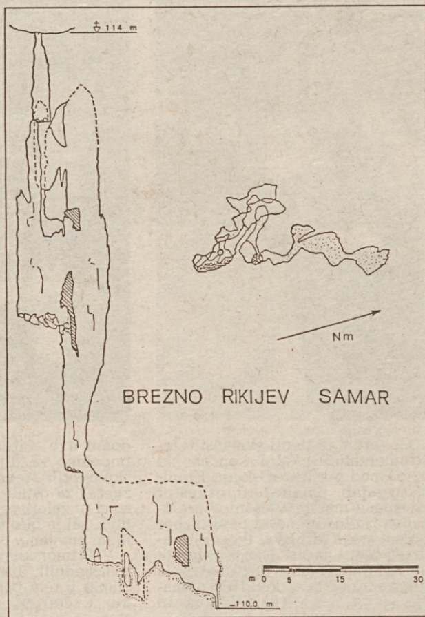
Prezrez in tloris brezna Rikijev Samar
