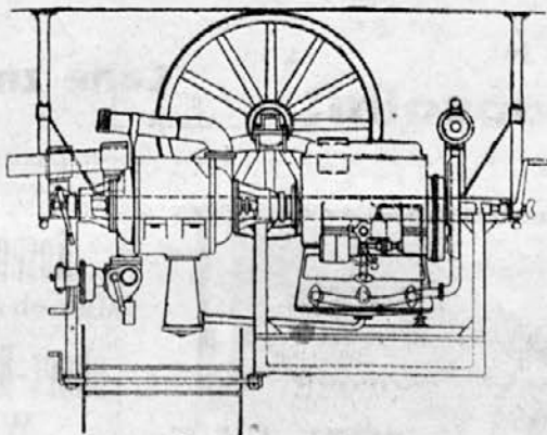
Motorna dvokolna brizgalnica z batnim brzotekim črpalom za visoki pritisek
