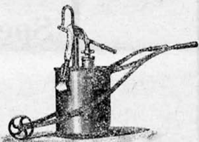
Vozna brenna točna brizgalnica, jednostavno brizgajoča.
