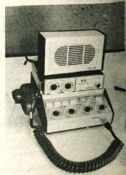
Najnovejši izdelek ISKRE: centralna postaja za občinske zveze RT-10-12/T
