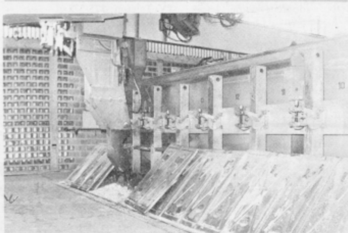
Prebijanje skorje v novi elektrolitski peči je povsem avtomatizirano in poteka z manevri iz premičnega dvigala. (Foto: M. Ozmeč.)
