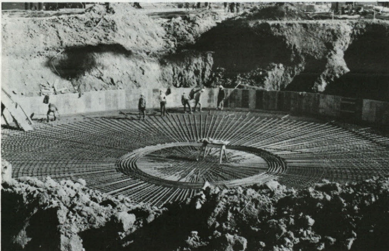
Kot da bi šlo za temelje raketne rampe - polaganje betonskega železa za temelj dimnika TEŠ IV.
