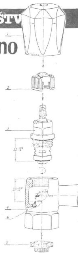
POZ.1 ROČAJ POZ.2 VMESNI ELEMENT POZ.3 BREZSUMNI VENTIL POZ.4 OHIŠJE ARMATURE POZ.5 TESNILO Z MREŽO POZ.6 SEDEŽ PIPE
