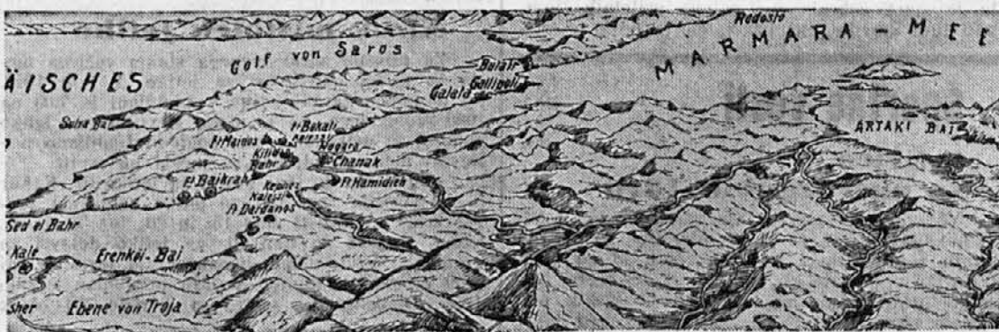
Celotni pogled na dardanelsko ožino, po morskem cestu iz Egejskega v Marmorsko morje.
